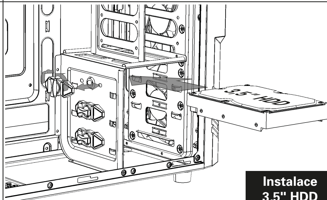
Instalace 3,5" jednotky
